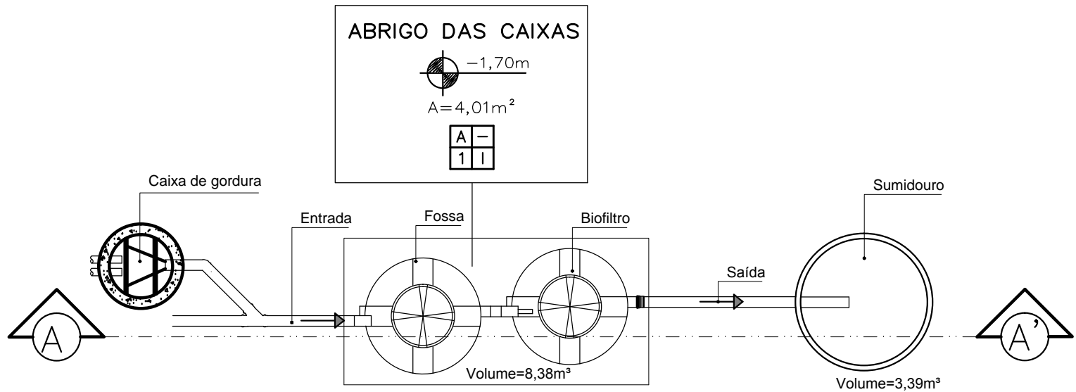
PLANTA BAIXA DO CONJUNTO
