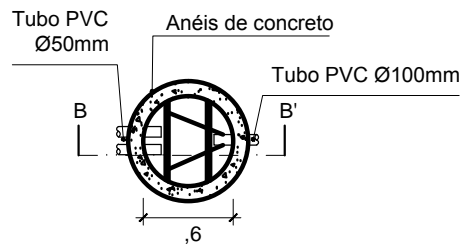
PLANTA BAIXA DA CAIXA DE GORDURA
