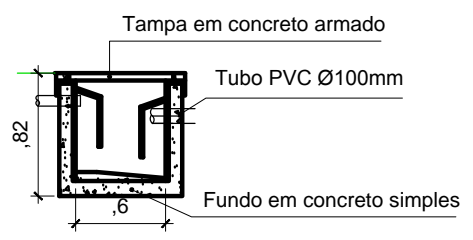
CORTE BB'
