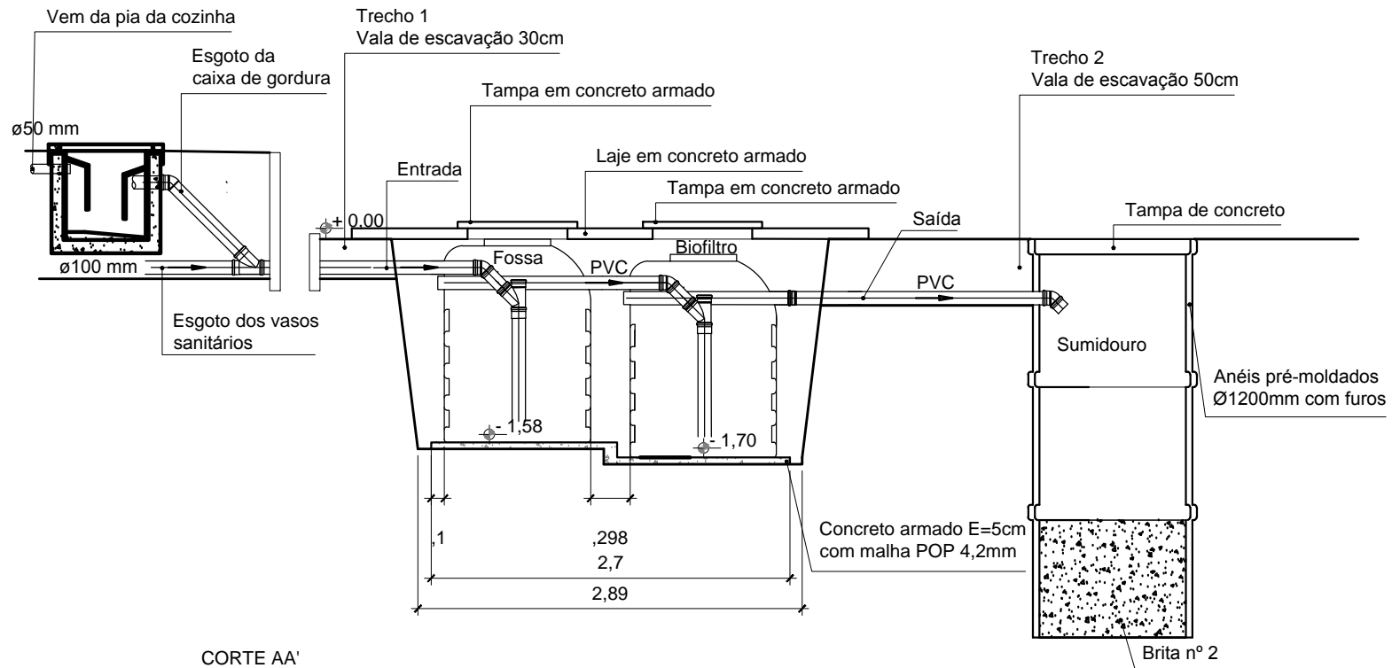
CORTE AA'
