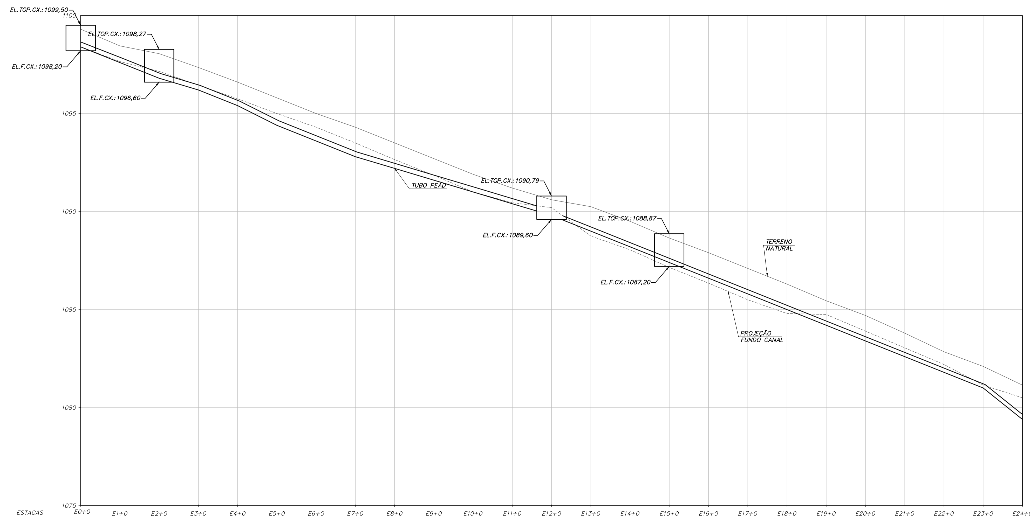
PERFIL LONGITUDINAL RAMAL 2 ESC. HORIZONTAL = 1:1000 VERTICAL = 1:100
