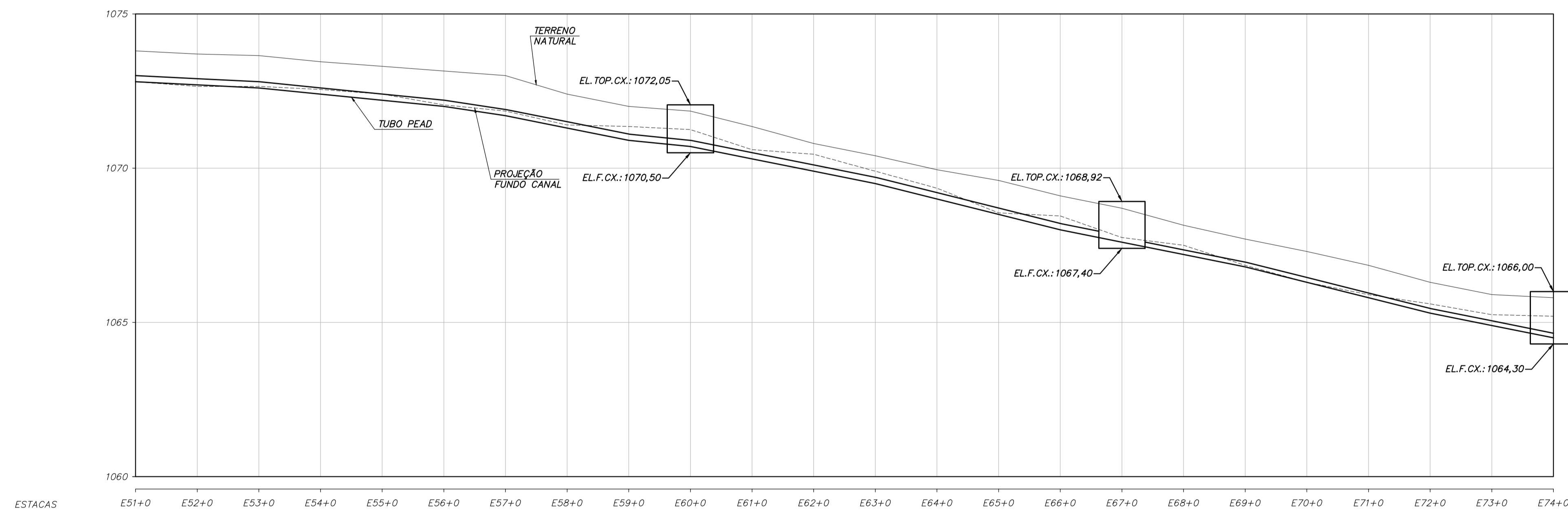
PERFIL LONGITUDINAL RAMAL 2 ESC. HORIZONTAL = 1:1000 ESC. VERTICAL = 1:100
