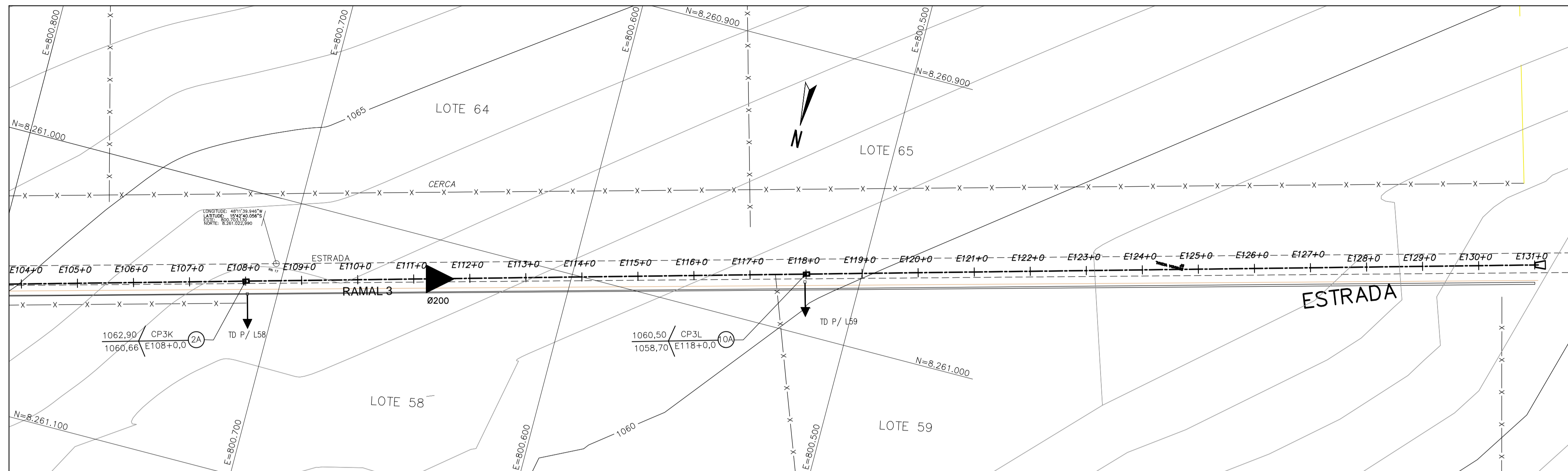
PLANTA - RAMAL 3 ESC: 1:1000
